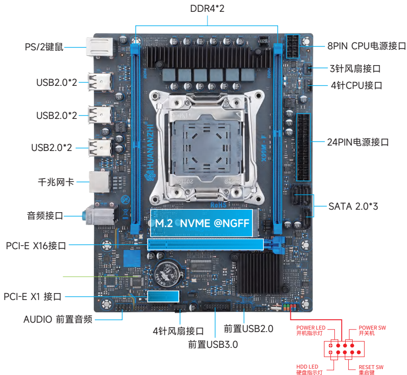
图1-1 X99M-F主板图解
