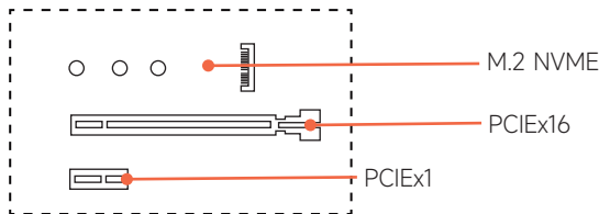
图2-3 PCI扩展插槽
