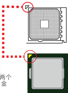
图2-7 CPU安装
